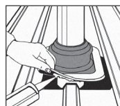
3. Naneste těsnící tmel.
