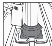
5. Manžetu upevněte pomocí samovrtných šroubů nebo rozpěrných trhacích nýtů.
