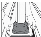
2. Manžetu vytvarujte podle profilu a obkreslete na plech.
