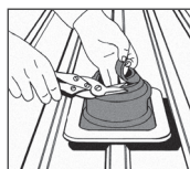
1. Manžetu přizpůsobte průměru potrubí.
